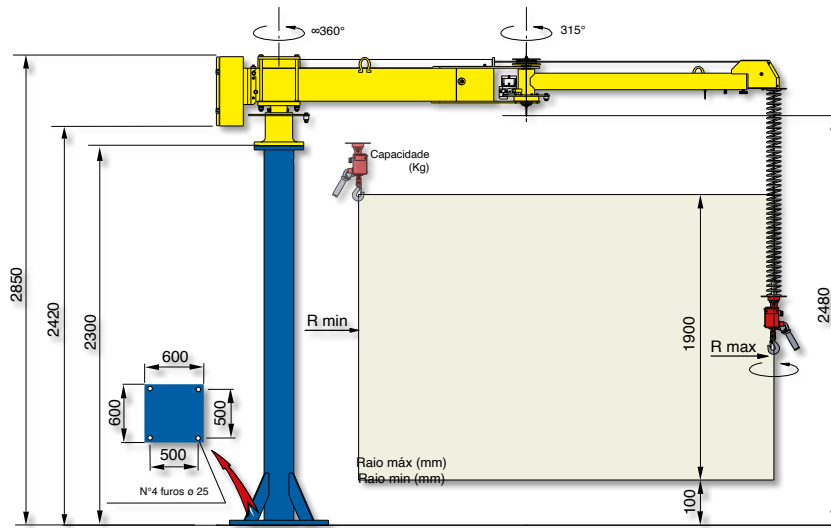
Versão estrutural: em base fixa, em base auto-estável oportunamente dimensionada.
